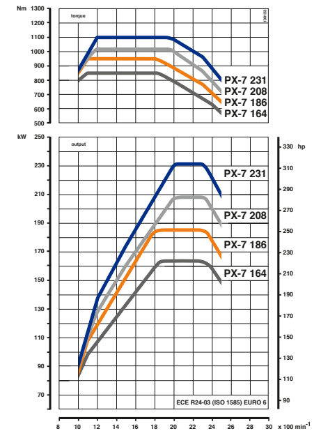
PACCAR PX-7
